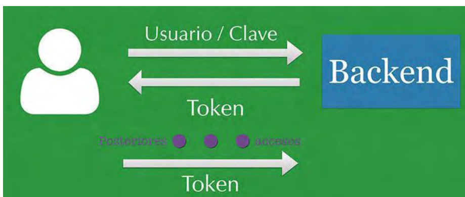
Fig. 2. Esquema conceptual de alto nivel del uso de Tokens en una API REST.
