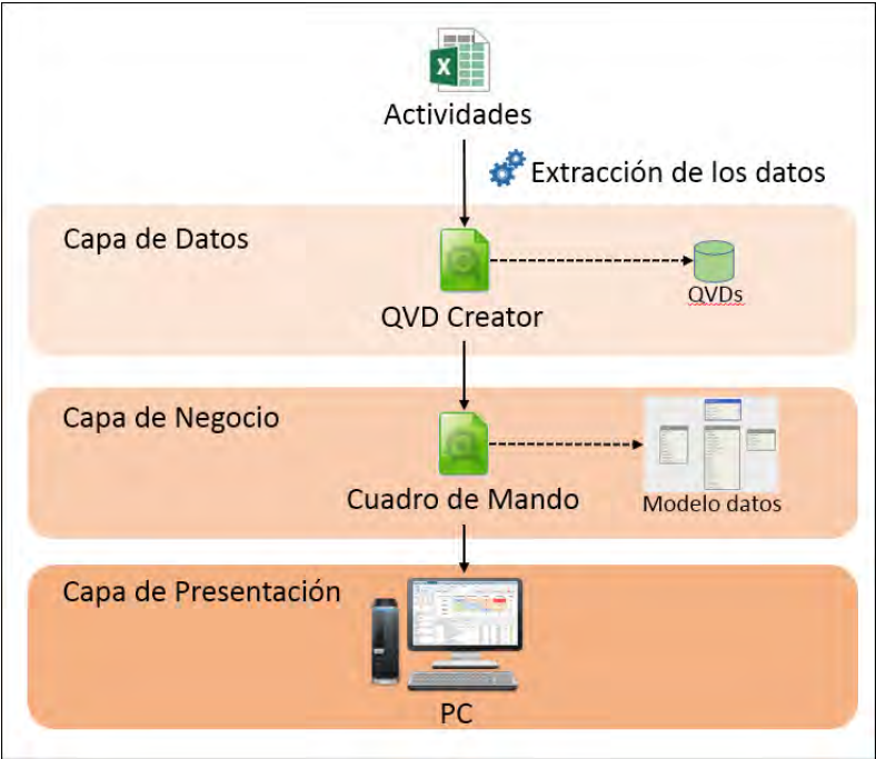
Fig. 1. Arquitectura de la solución
